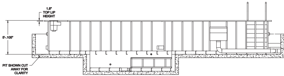
ELEVATION
