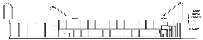
ELEVATION
